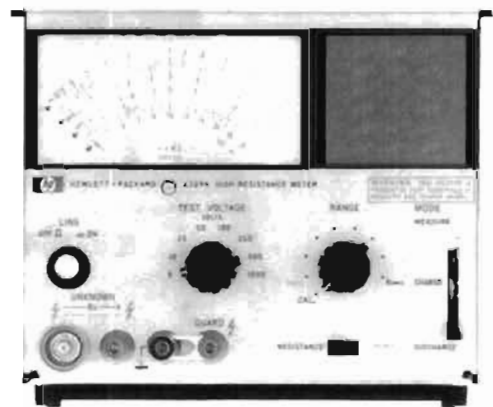
HP 4329A
